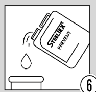
Шаг 6 - Пассивация
